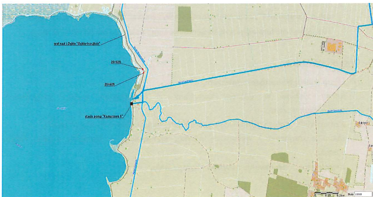
Plan sytuacyjny 2 Wał nad Jeziorem Dąbie „Dąbie-Inoujście” w km 18+609÷20+420
